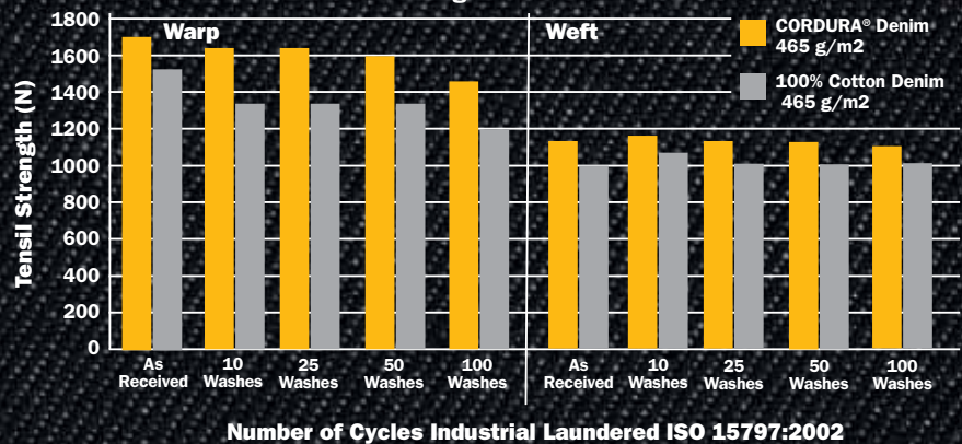
CORDURA ® Denim fabric vs 100% Cotton Denim fabric Tensile Strength BS EN ISO 13934-1:1999
