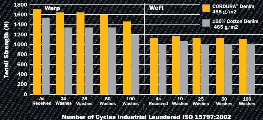
CORDURA® Denim fabric vs 100% Cotton Denim fabric Tensile Strength BS EN ISO 13934-1:1999
